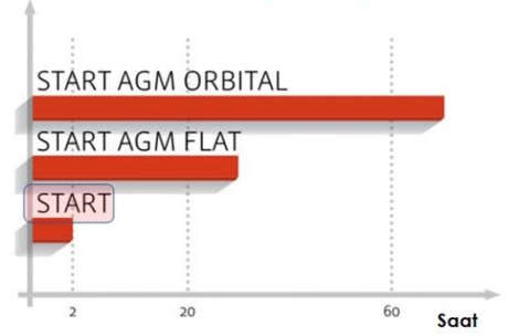
START & START AGM Titreşim Direnci (6G / 35Hz)
