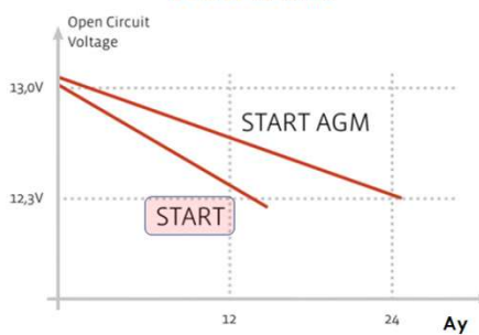
START & START AGM 20°C'de Raf Ömrü
